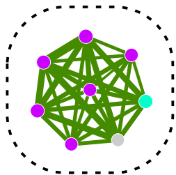
module6 (p.value=3.23e-03)
