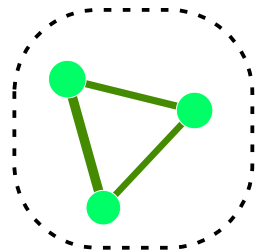
module8 (p.value=5.14e-03)
