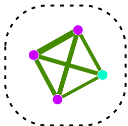
module9 (p.value=5.24e-03)
