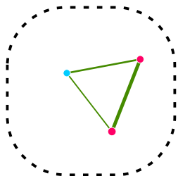
module13 (p.value=8.55e-03)
