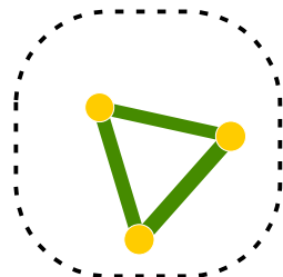
module8 (p.value=5.14e-03)
