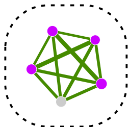
module6 (p.value=3.23e-03)
